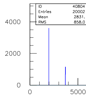
40ns.TDC.1290.sl.08.ch.03
