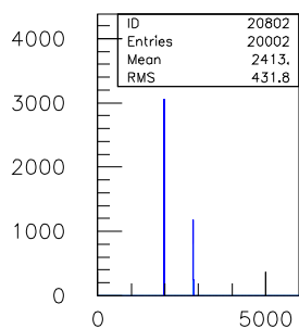
20ns.TDC.1290.sl.08.ch.01
