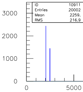
10ns.TDC.1290.sl.09.ch.10
