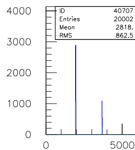
40ns.TDC.1290.sl.07.ch.06
