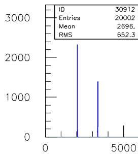
30ns.TDC.1290.sl.09.ch.11
