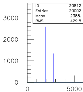
20ns.TDC.1290.sl.08.ch.11
