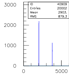
40ns.TDC.1290.sl.09.ch.08
