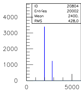
20ns.TDC.1290.sl.08.ch.03
