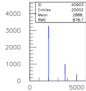
40ns.TDC.1290.sl.09.ch.02
