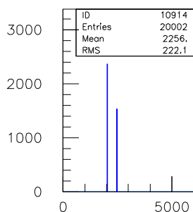
10ns.TDC.1290.sl.09.ch.13
