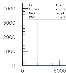
40ns.TDC.1290.sl.07.ch.05
