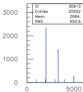
30ns.TDC.1290.sl.09.ch.12
