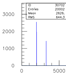
30ns.TDC.1290.sl.07.ch.01
