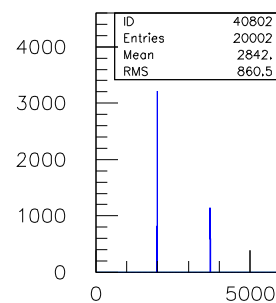
40ns.TDC.1290.sl.08.ch.01
