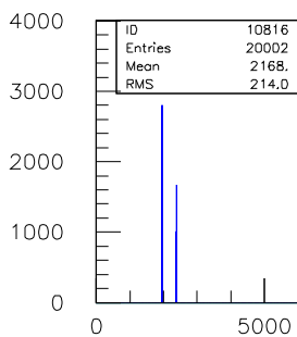
10ns.TDC.1290.sl.08.ch.15
