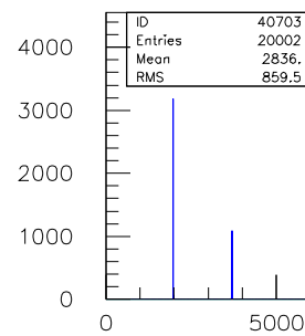
40ns.TDC.1290.sl.07.ch.02
