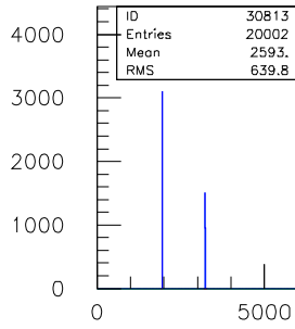
30ns.TDC.1290.sl.08.ch.12
