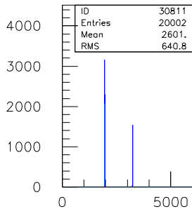
30ns.TDC.1290.sl.08.ch.10
