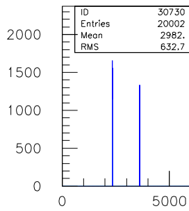
30ns.TDC.1290.sl.07.ch.29
