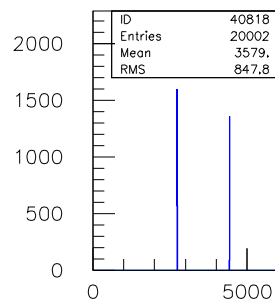
40ns.TDC.1290.sl.08.ch.17
