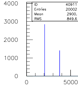
40ns.TDC.1290.sl.09.ch.10
