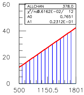
TDC.1290.sl.10.ch.00
