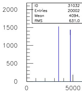
30ns.TDC.1290.sl.10.ch.31
