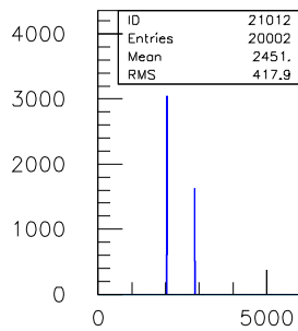
20ns.TDC.1290.sl.10.ch.11
