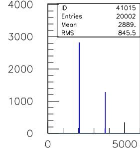
40ns.TDC.1290.sl.10.ch.14
