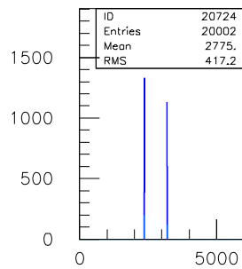
20ns.TDC.1290.sl.07.ch.23
