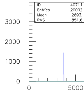
40ns.TDC.1290.sl.07.ch.10
