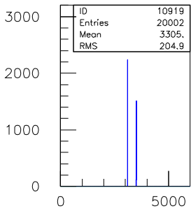
10ns.TDC.1290.sl.09.ch.18
