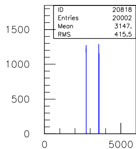
20ns.TDC.1290.sl.08.ch.17
