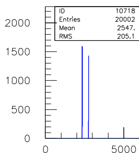
10ns.TDC.1290.sl.07.ch.17
