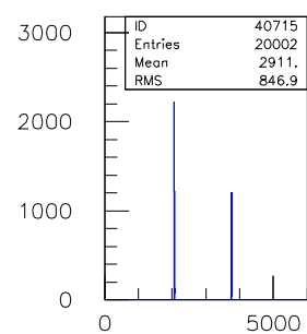
40ns.TDC.1290.sl.07.ch.14
