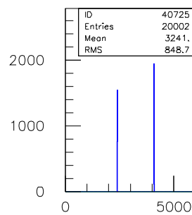
40ns.TDC.1290.sl.07.ch.24
