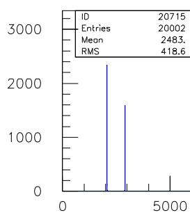
20ns.TDC.1290.sl.07.ch.14
