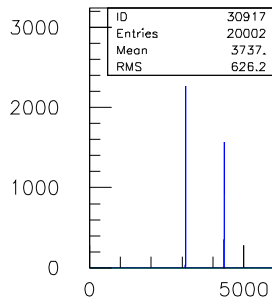
30ns.TDC.1290.sl.09.ch.16
