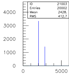
20ns.TDC.1290.sl.10.ch.02
