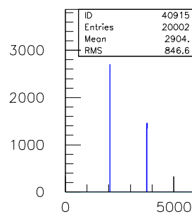
40ns.TDC.1290.sl.09.ch.14
