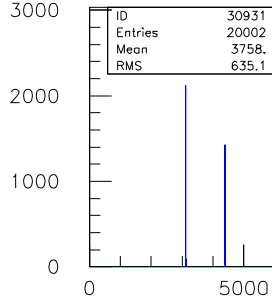
30ns.TDC.1290.sl.09.ch.30
