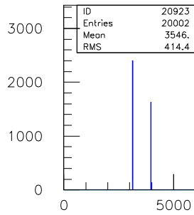
20ns.TDC.1290.sl.09.ch.22
