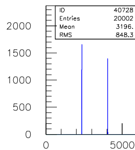
40ns.TDC.1290.sl.07.ch.27
