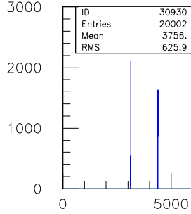
30ns.TDC.1290.sl.09.ch.29
