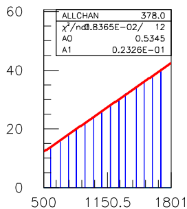
TDC.1290.sl.08.ch.02
