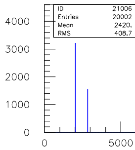
20ns.TDC.1290.sl.10.ch.05
