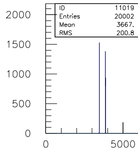
10ns.TDC.1290.sl.10.ch.18
