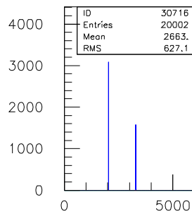
30ns.TDC.1290.sl.07.ch.15
