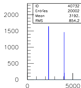
40ns.TDC.1290.sl.07.ch.31
