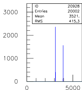
20ns.TDC.1290.sl.09.ch.27
