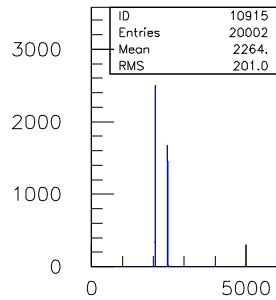
10ns.TDC.1290.sl.09.ch.14
