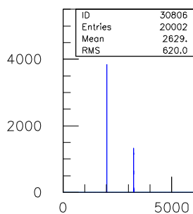
30ns.TDC.1290.sl.08.ch.05
