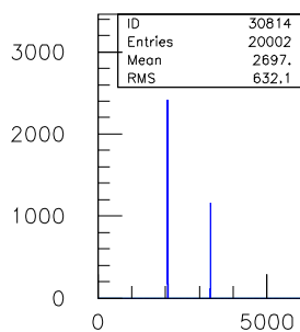
30ns.TDC.1290.sl.08.ch.13
