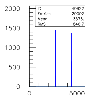
40ns.TDC.1290.sl.08.ch.21
