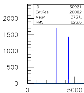
30ns.TDC.1290.sl.09.ch.20
