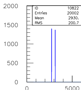
10ns.TDC.1290.sl.08.ch.21
