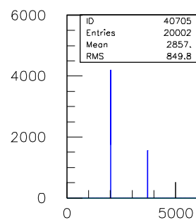
40ns.TDC.1290.sl.07.ch.04
