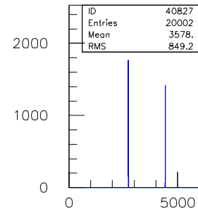
40ns.TDC.1290.sl.08.ch.26
