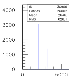
30ns.TDC.1290.sl.09.ch.05
