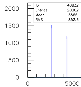
40ns.TDC.1290.sl.08.ch.31
