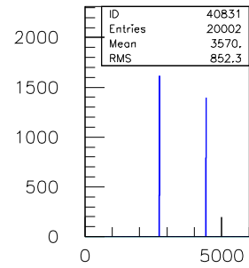
40ns.TDC.1290.sl.08.ch.30
