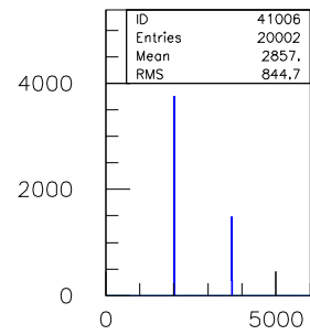
40ns.TDC.1290.sl.10.ch.05
