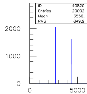
40ns.TDC.1290.sl.08.ch.19
