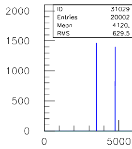
30ns.TDC.1290.sl.10.ch.28
