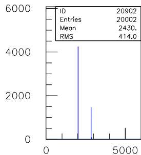
20ns.TDC.1290.sl.09.ch.01
