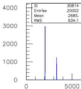
30ns.TDC.1290.sl.08.ch.13
