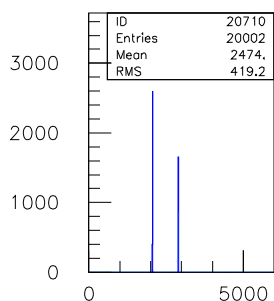
20ns.TDC.1290.sl.07.ch.09
