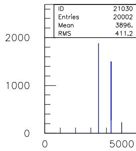
20ns.TDC.1290.sl.10.ch.29
