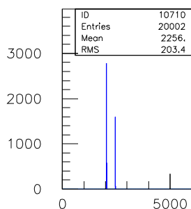
10ns.TDC.1290.sl.07.ch.09
