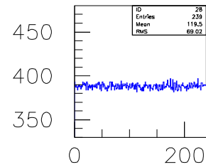
FADC BaseLine
