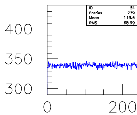
FADC BaseLine
